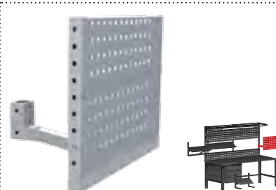
perforiran panel MTP: izrezi 10 x 10 mm, raster 38 mm, primeren za držala za orodje QDN
