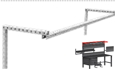
ogrodje za montažo luči MTO: montira se na panel MTR, primerno za namestitev luči ELE_OSV_xx, stojalo dolžine 2000 mm ima na sredini prečko
